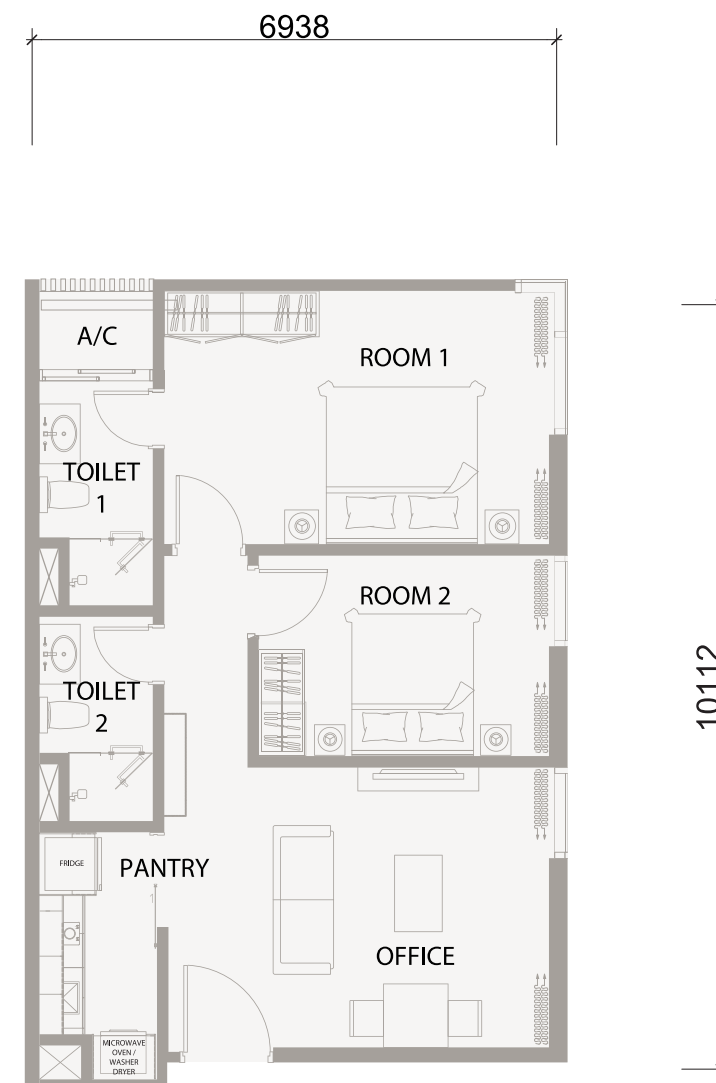
户型 LH 775ft 2 (平方尺) 71.99m 2 (平方米)
